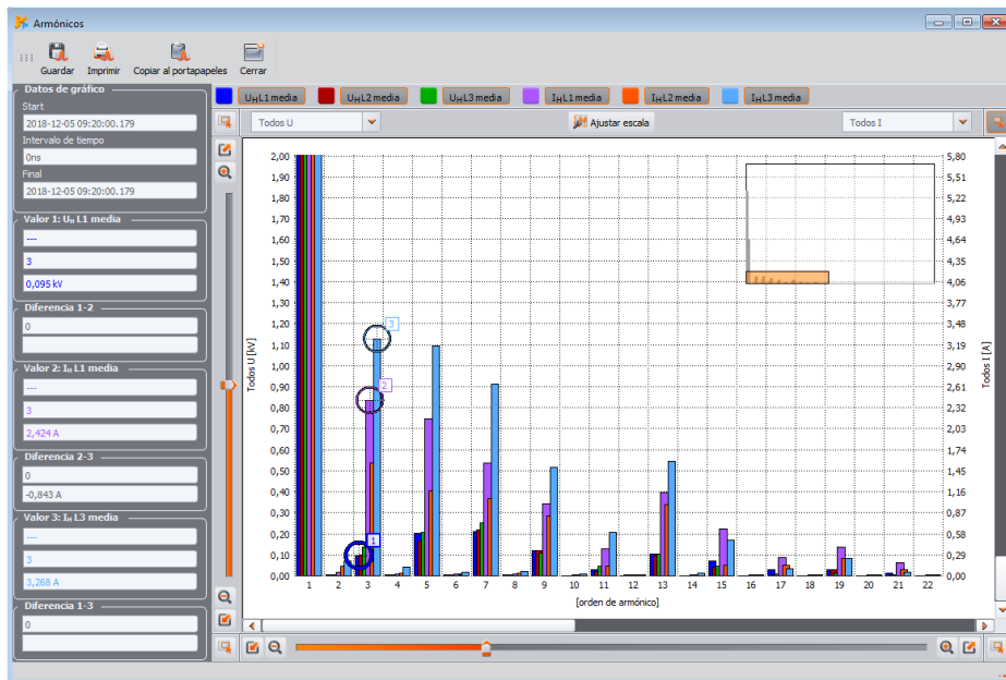
Fig. 61. Gráfico de armónicos.
