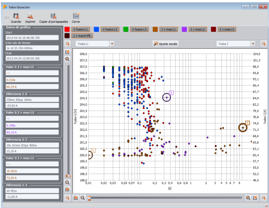
Fig. 70. Análisis de eventos - diagrama de valor/ duración.
