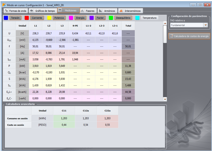
Fig. 48. Indicaciones de los valores físicos y sumarios.
