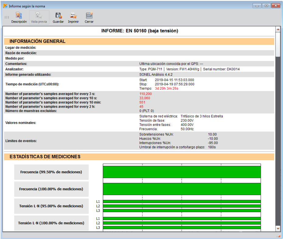
Fig. 65. Informe de medición del cumplimiento con la norma EN 50160.
