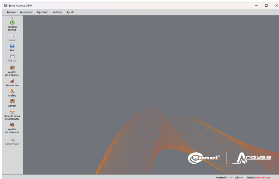
Fig. 5. Pantalla principal.
