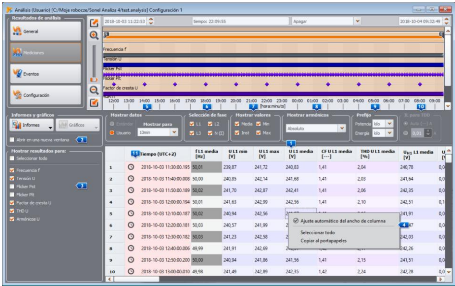
Fig. 58. Ventana Mediciones.
