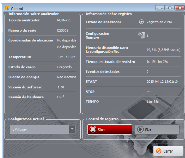
Fig. 75. Ventana Control.
