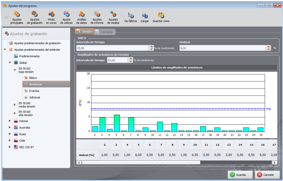
Fig. 79. Registro según EN 50160 - ajustes de armónicos.
