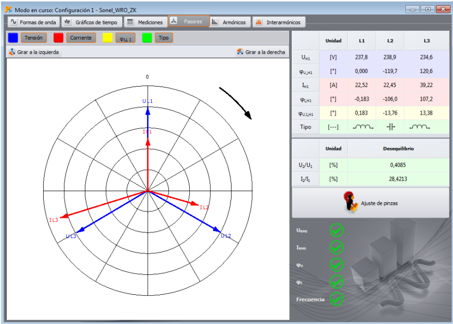
Fig. 49. Diagrama fasorial para conexin en estrella.
