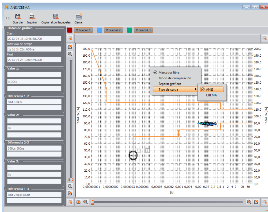
Fig. 71. Diagrama ANSI/CBEMA.
