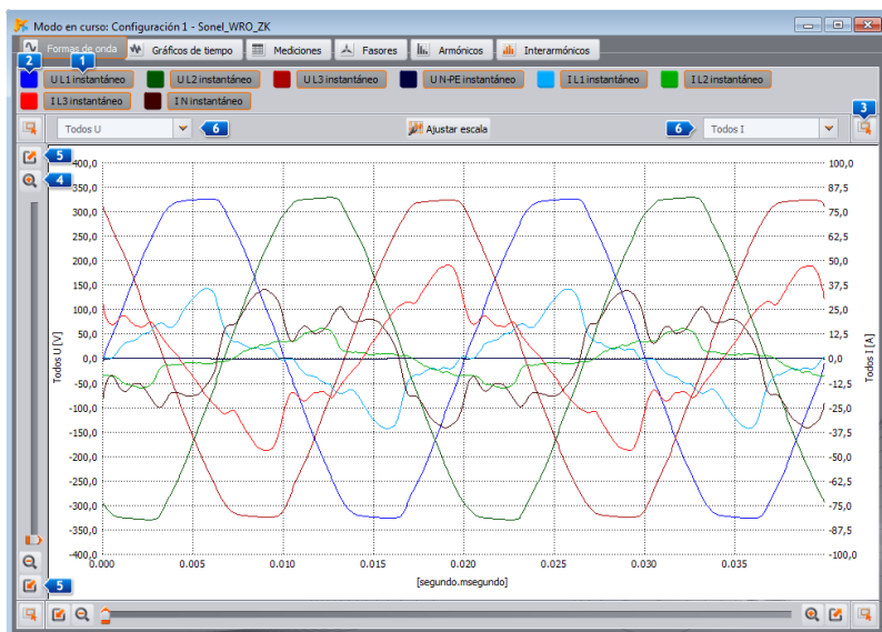
Fig. 45. La pantalla en el modo de lectura de los datos actuales - formas de onda.
