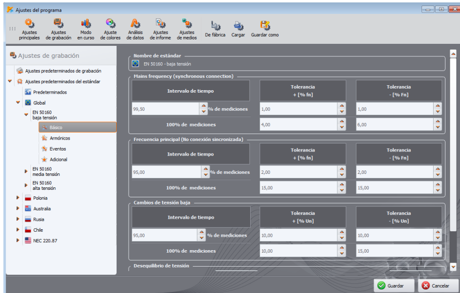
Fig. 78. Registro según la norma - ajustes básicos.
