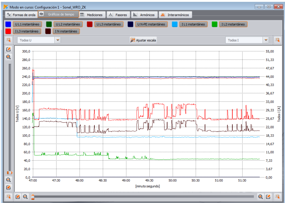
Fig. 47. Diagrama de valores en tiempo real.
