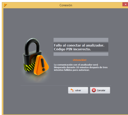
Fig. 9. PIN incorrecto.
