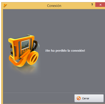
Fig. 10. Conexión perdida.
