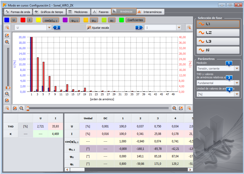
Fig. 50. Armónicos.
