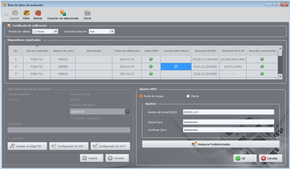
Fig. 42. Pantalla de configuración de Wi-Fi en modo online (modo de punto de acceso en el analizador).
