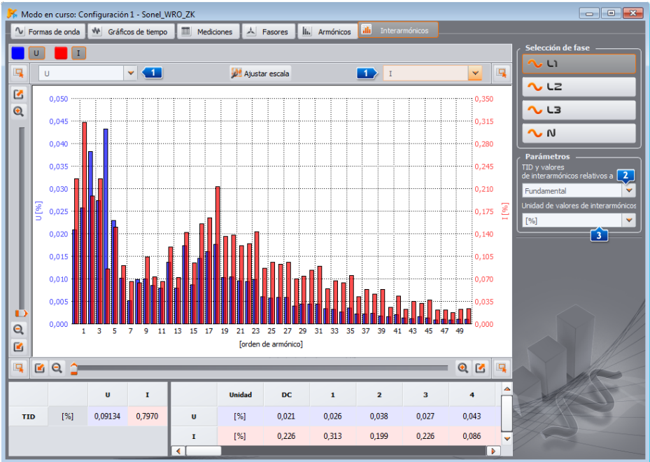
Fig. 52. Diagrama de interarmónicos.
