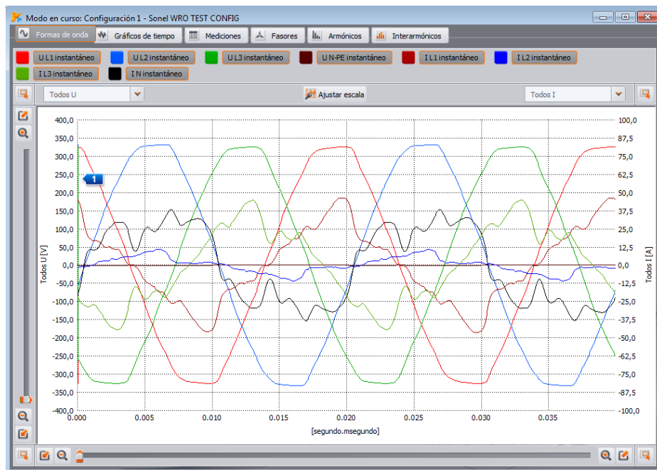
Fig. 46. La sincronización de formas de onda entre diferentes analizadores: se ve el marcador de sincronización con el tiempo GPS.
