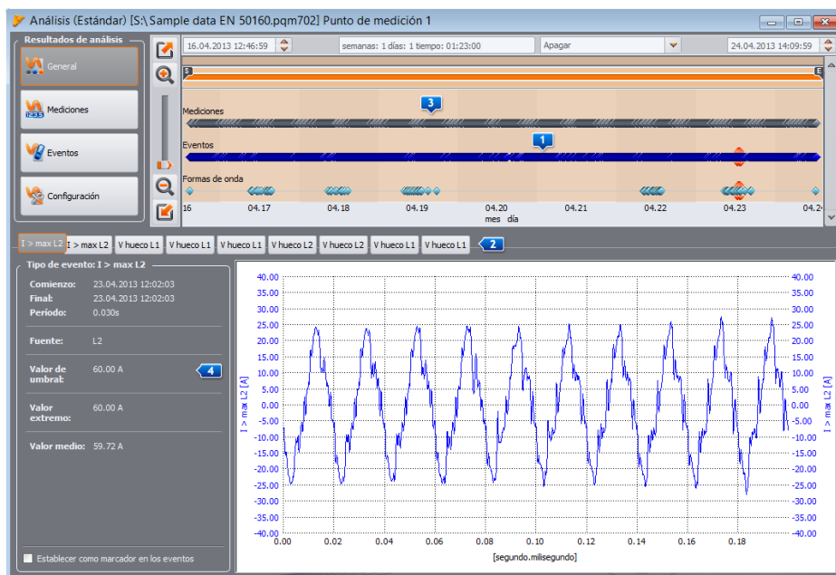
Fig. 57. Ventana general con la vista previa de la forma de onda.
