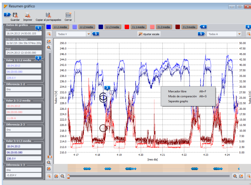
Fig. 60. Ventana del gráfico de tiempos.
