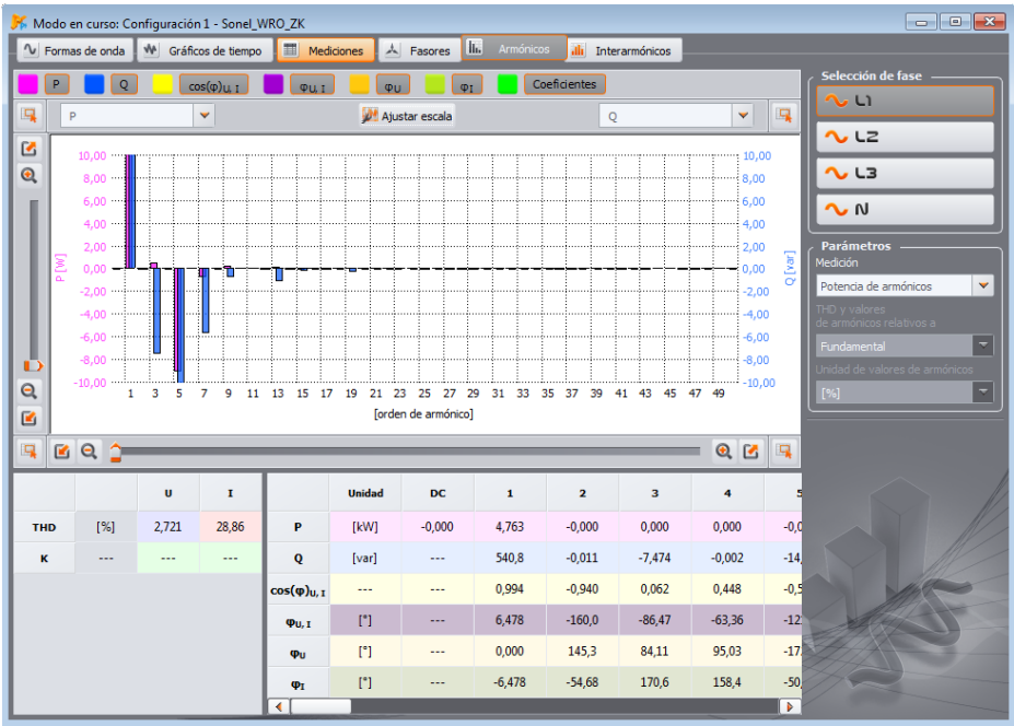
Fig. 51. La pantalla con las potencias de armónicos.
