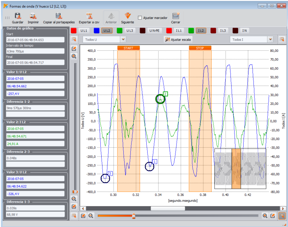
Fig. 72. Gráfico con la forma de onda inicial y final.
